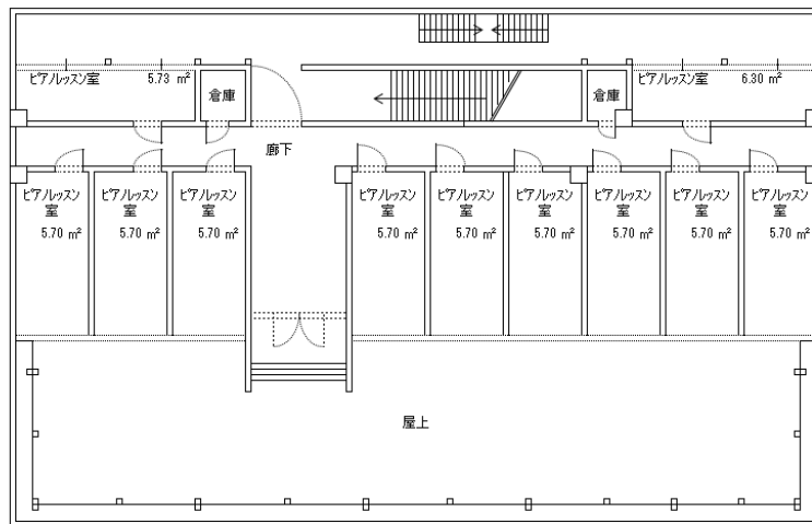
5 階 平 面 図
