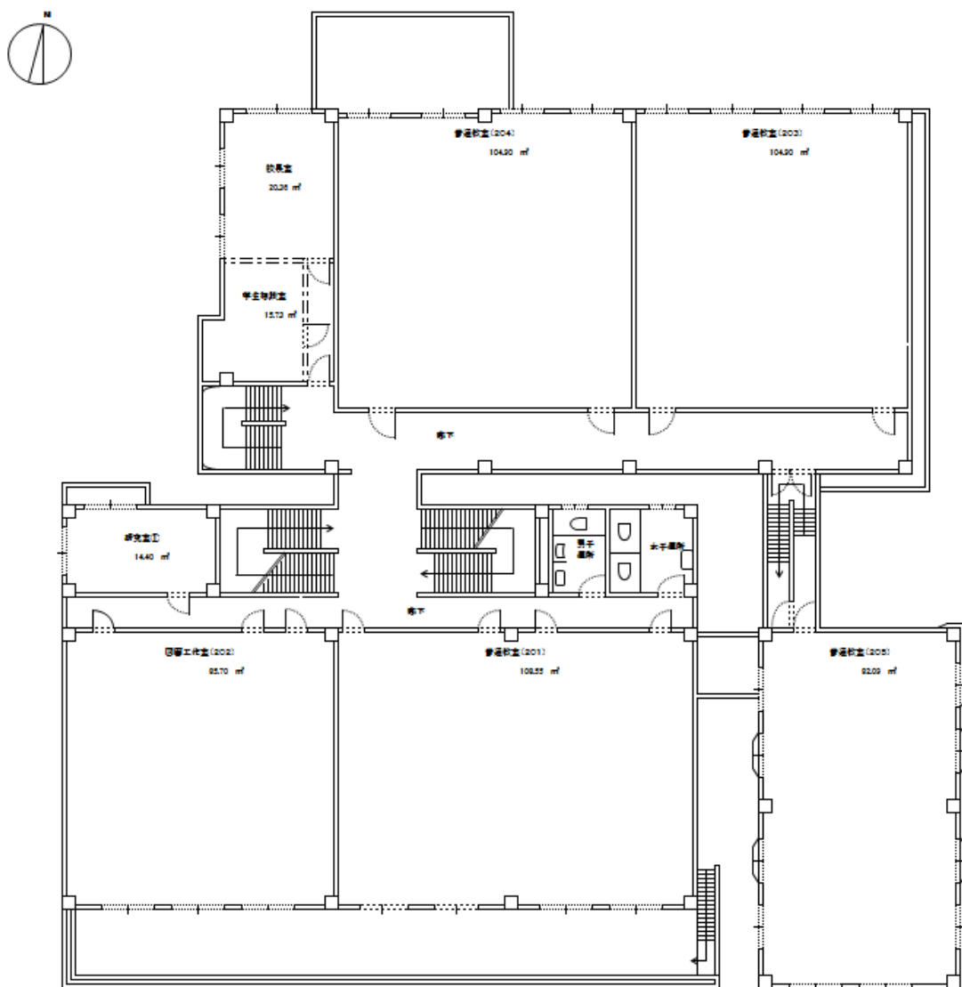
2 階 平 面 图
