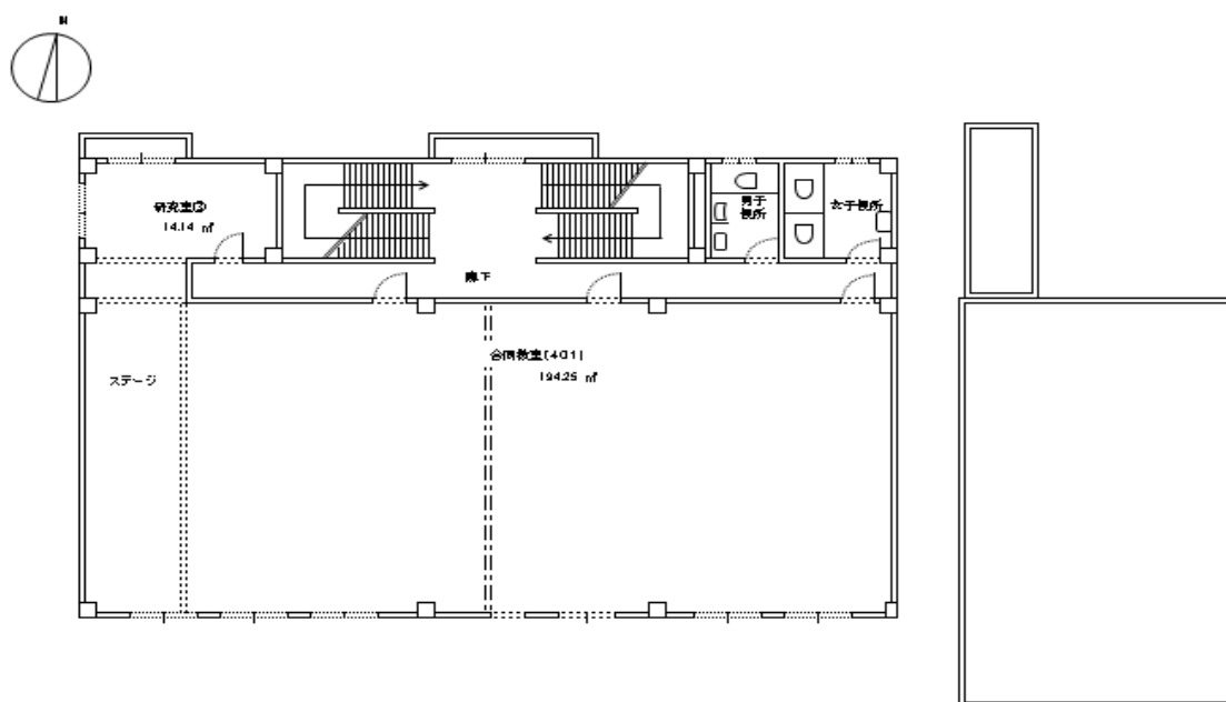
4 階 平 面 図
