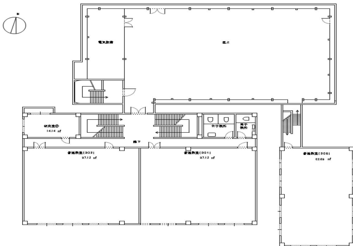
3 階 平 面 図
